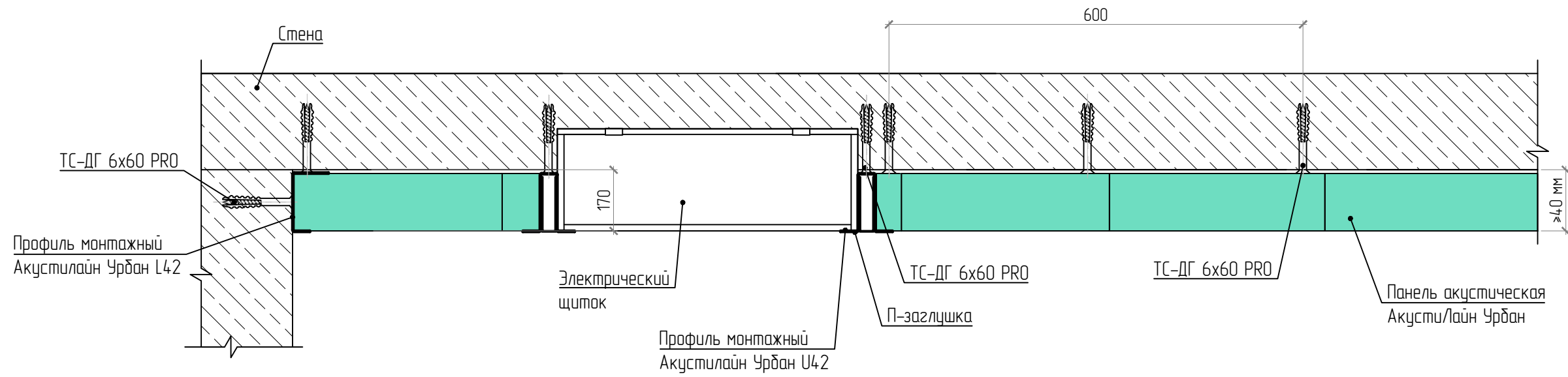
Разрез 4-4
