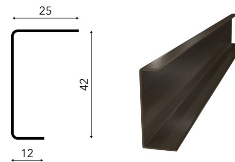
AKUSTILINE URBAN L42
