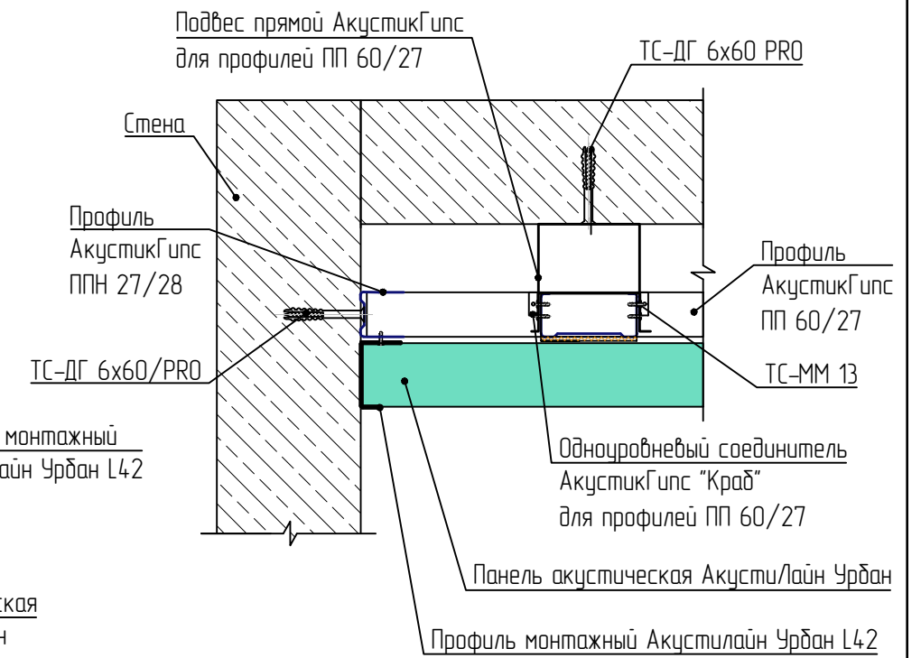
Оформление внутреннего угла. Горизонтальный разрез
