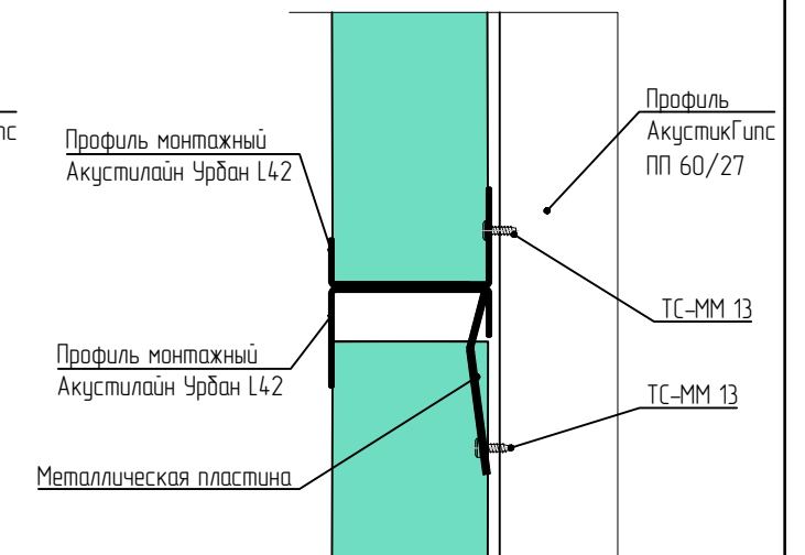
Узел 6 (Вариант 3)
