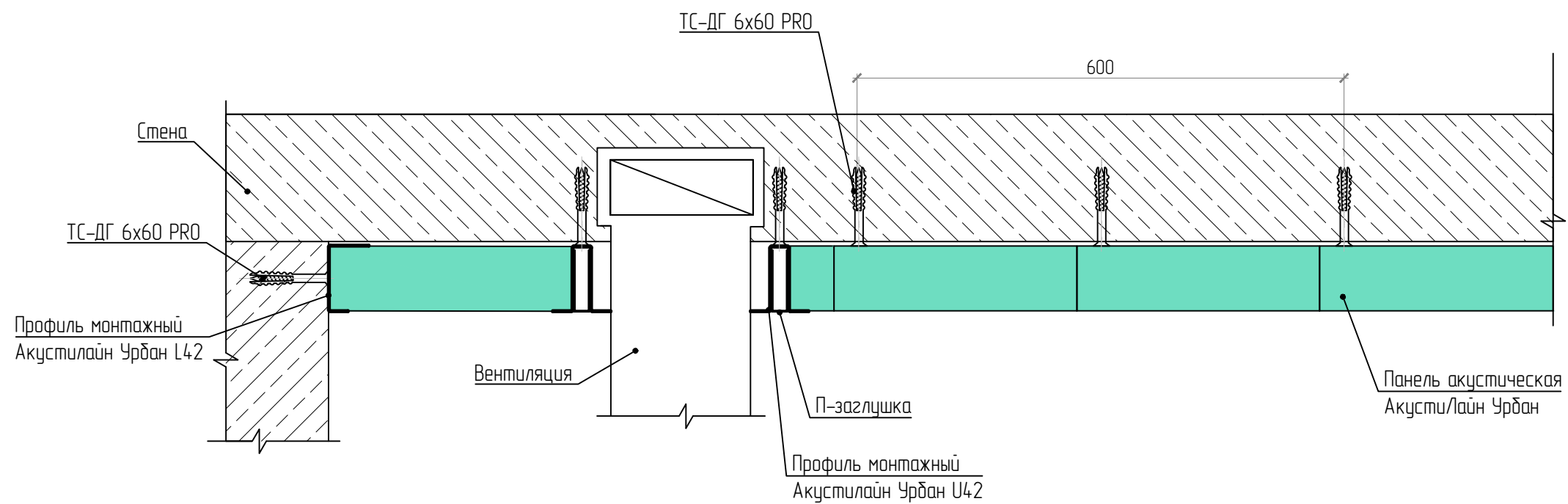
Разрез 5-5
