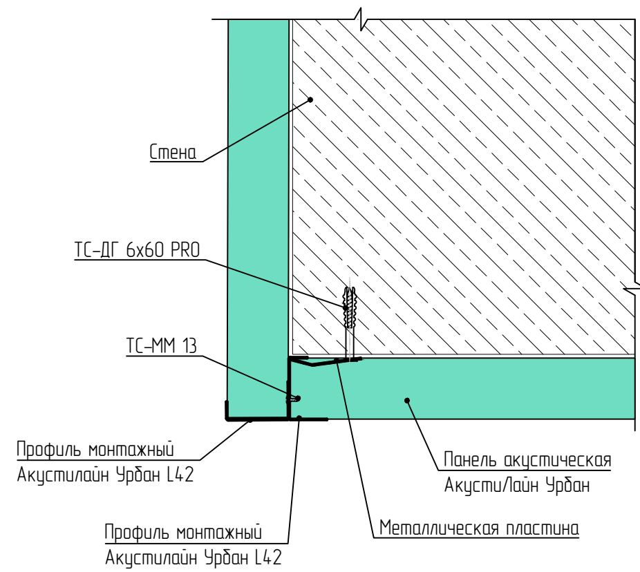
Оформление внешнего угла. Вариант 1 Горизонтальный разрез
