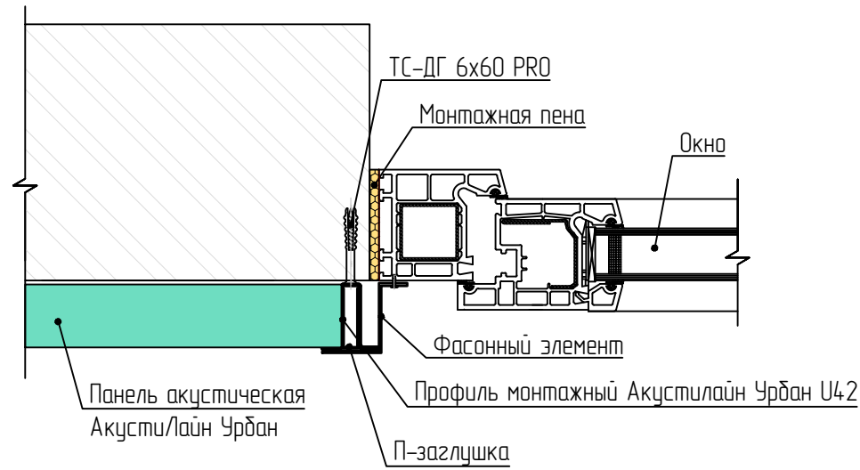
Узел оконного откоса. Горизонтальный разрез
