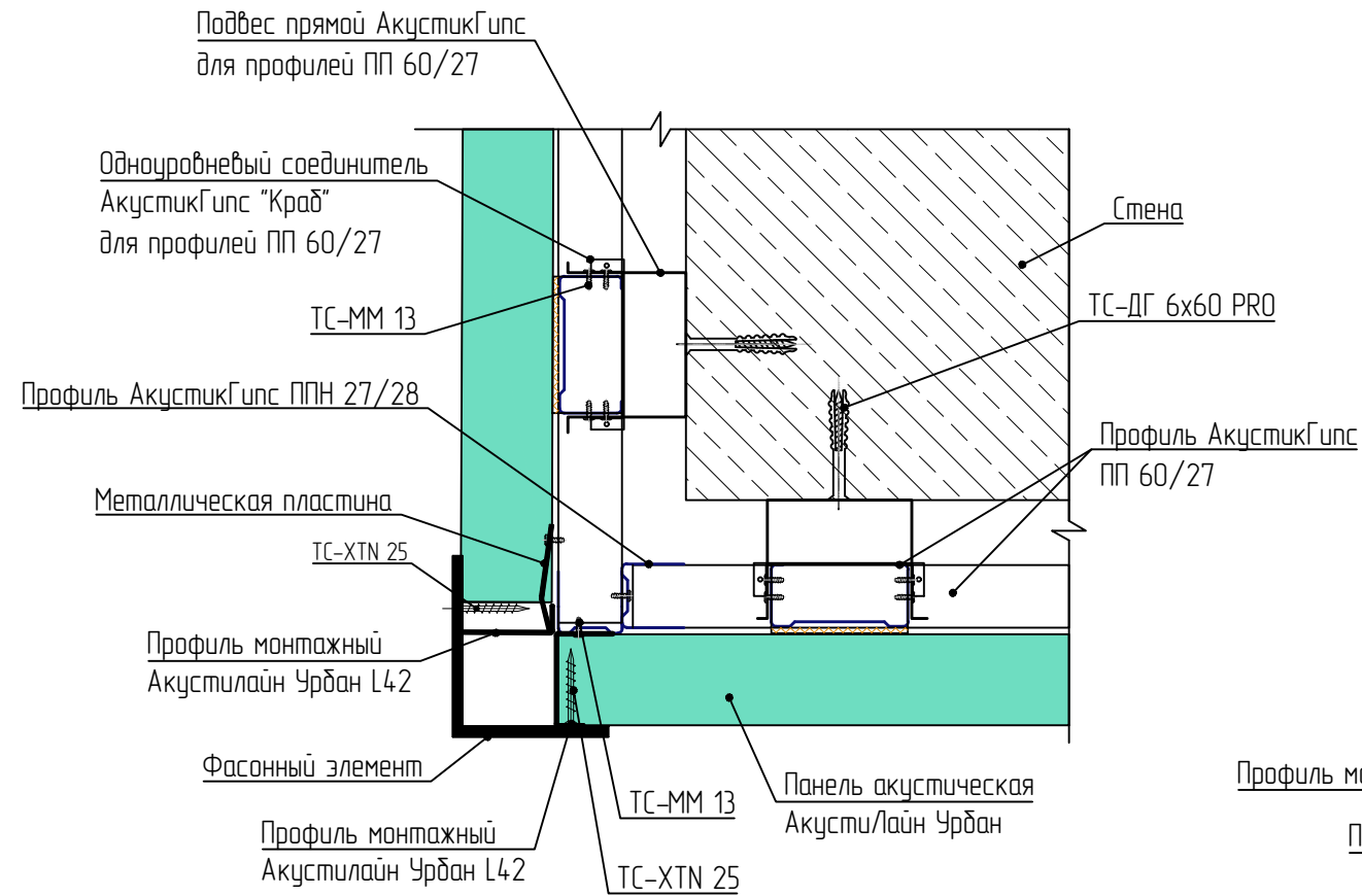
Оформление внешнего угла. Вариант 1 Горизонтальный разрез
