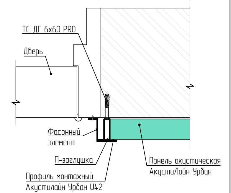
Примыкание панели к дверной конструкции. Горизонтальный разрез
