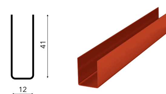
П-ЗАГЛУШКА К ПРОФИЛЮ МОНТАЖНОМУ AKUSTILINE U42
