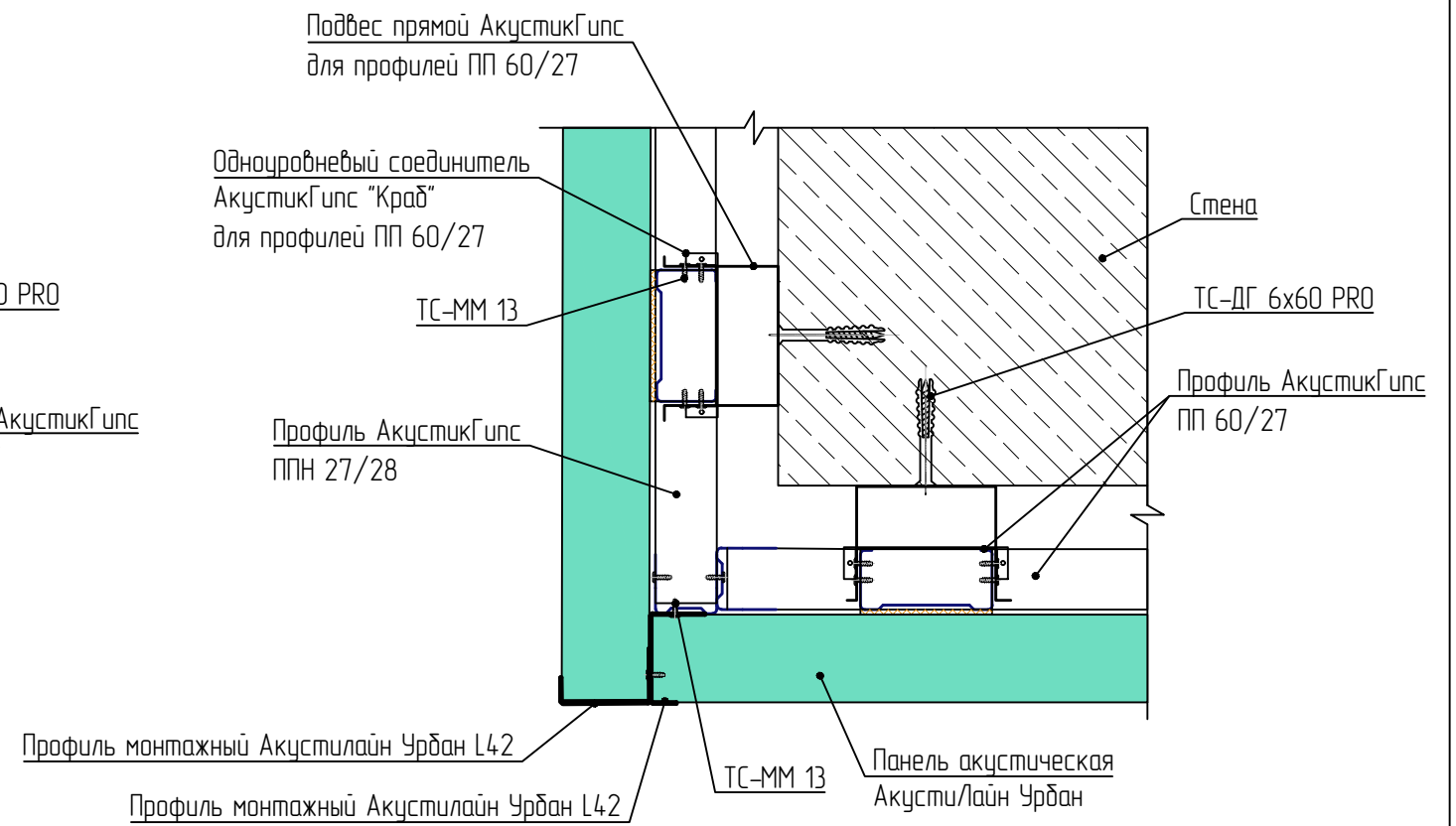
Оформление внешнего угла. Вариант 2 Горизонтальный разрез
