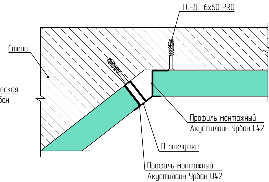
Оформление внутреннего угла >90°. Горизонтальный разрез
