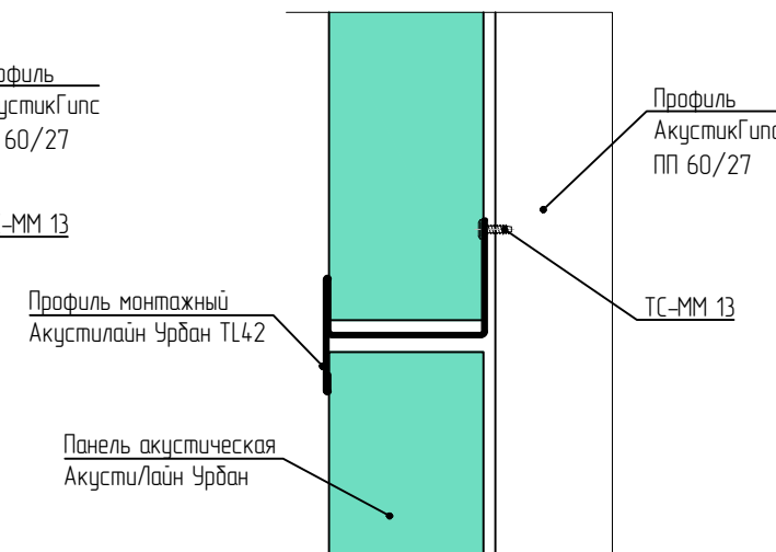
Узел 6 (Вариант 2)
