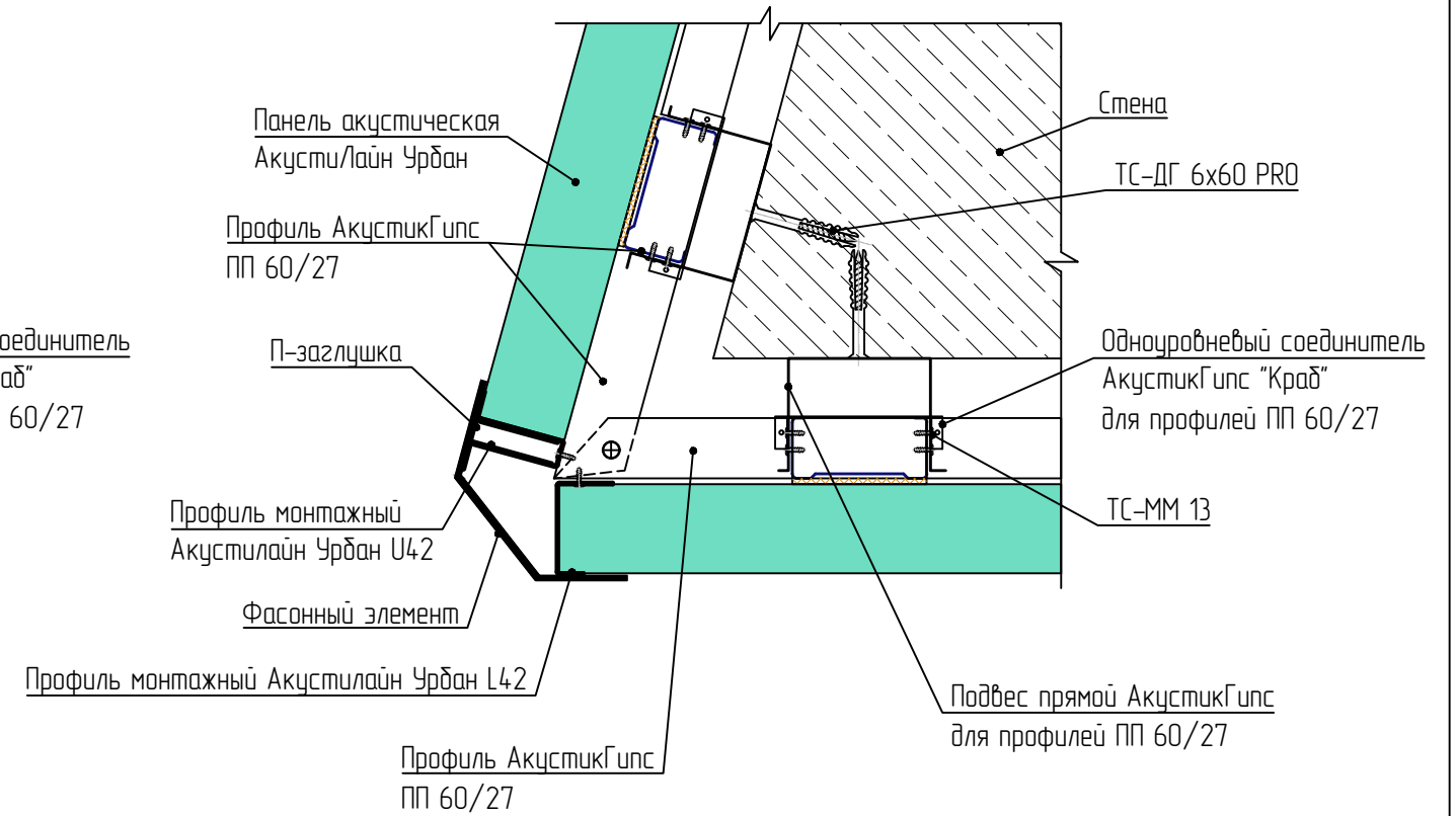
Оформление внешнего угла < 90°. Горизонтальный разрез
