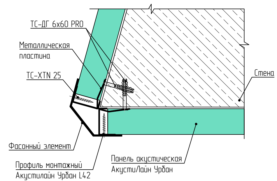
Оформление внешнего угла <90° Горизонтальный разрез
