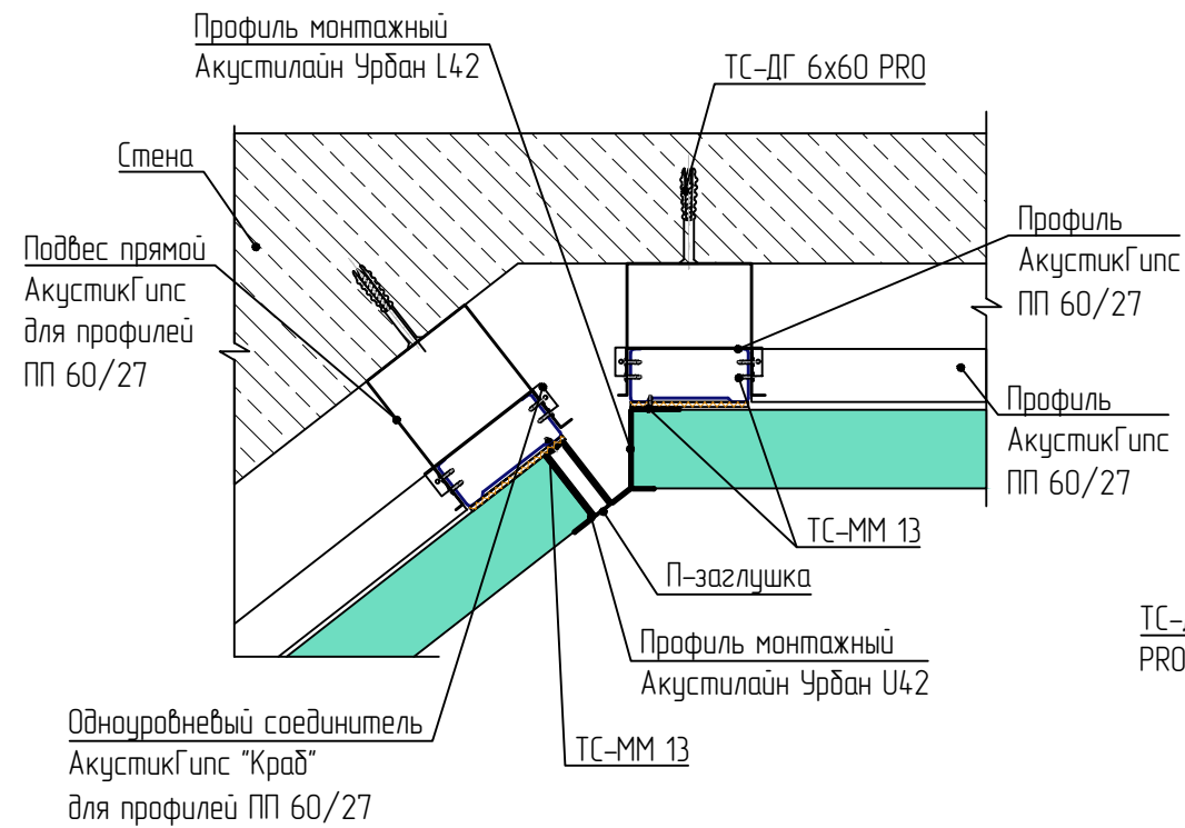
Оформление внутреннего угла >90^\circ . Горизонтальный разрез
