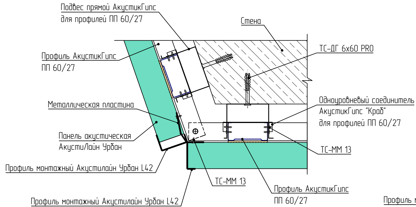
Оформление внешнего угла > 90°. Горизонтальный разрез
