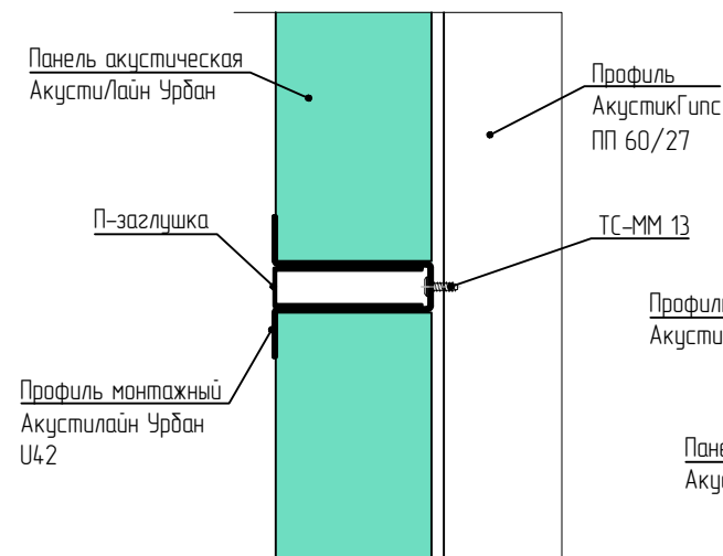
Узел 6 (Вариант 1)
